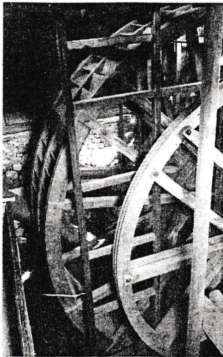
Das hölzerne Kehrrad – ein technisches Denkmal.
