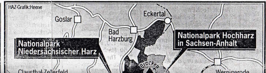
Auch die vom sauren Regen zerstörten Waldgebiete auf dem Bruchberg sind Bestandteil des Nationalparks Harz.
