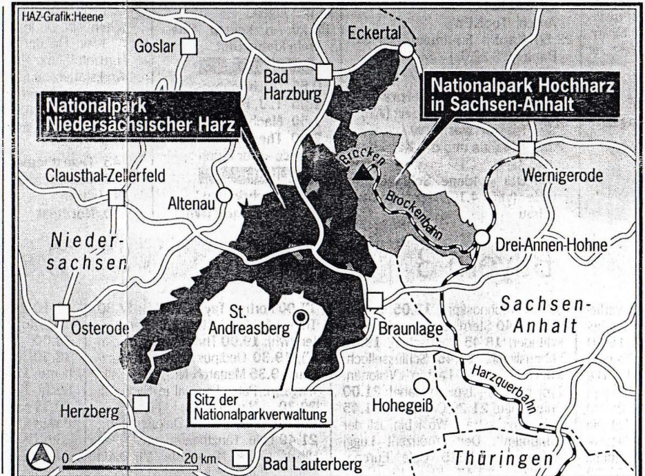
Auch die vom sauren Regen zerstörten Waldgebiete auf dem Bruchberg sind Bestandteil des Nationalparks Harz.
